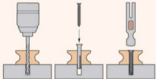
Předvrtaný otvor \varnothing 6mm Natloukací hmoždinka 6 x 80mm (hranol 40mm)
